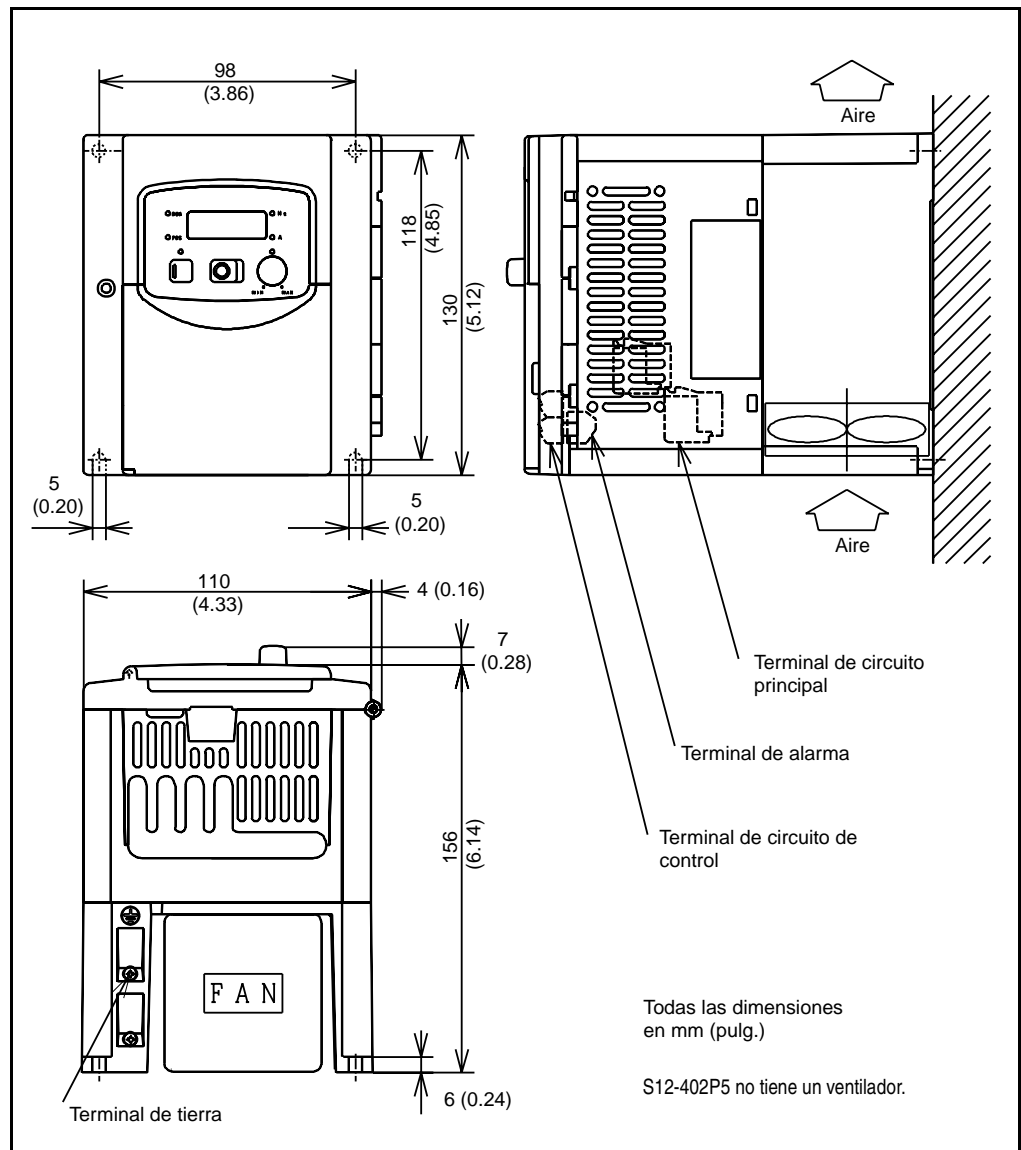
Figura A.7 – Dimensiones del S12-402P5/403P8/405P5
