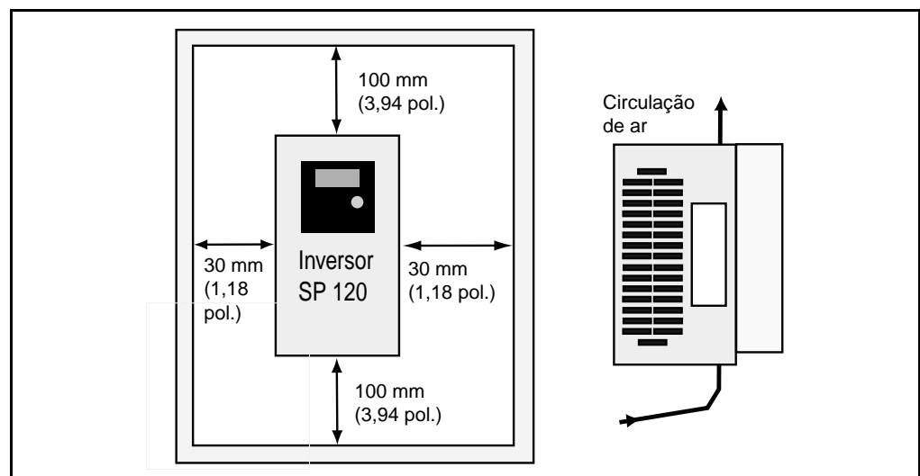
Figura 2.1 – Distâncias mínimas para a circulação de ar
