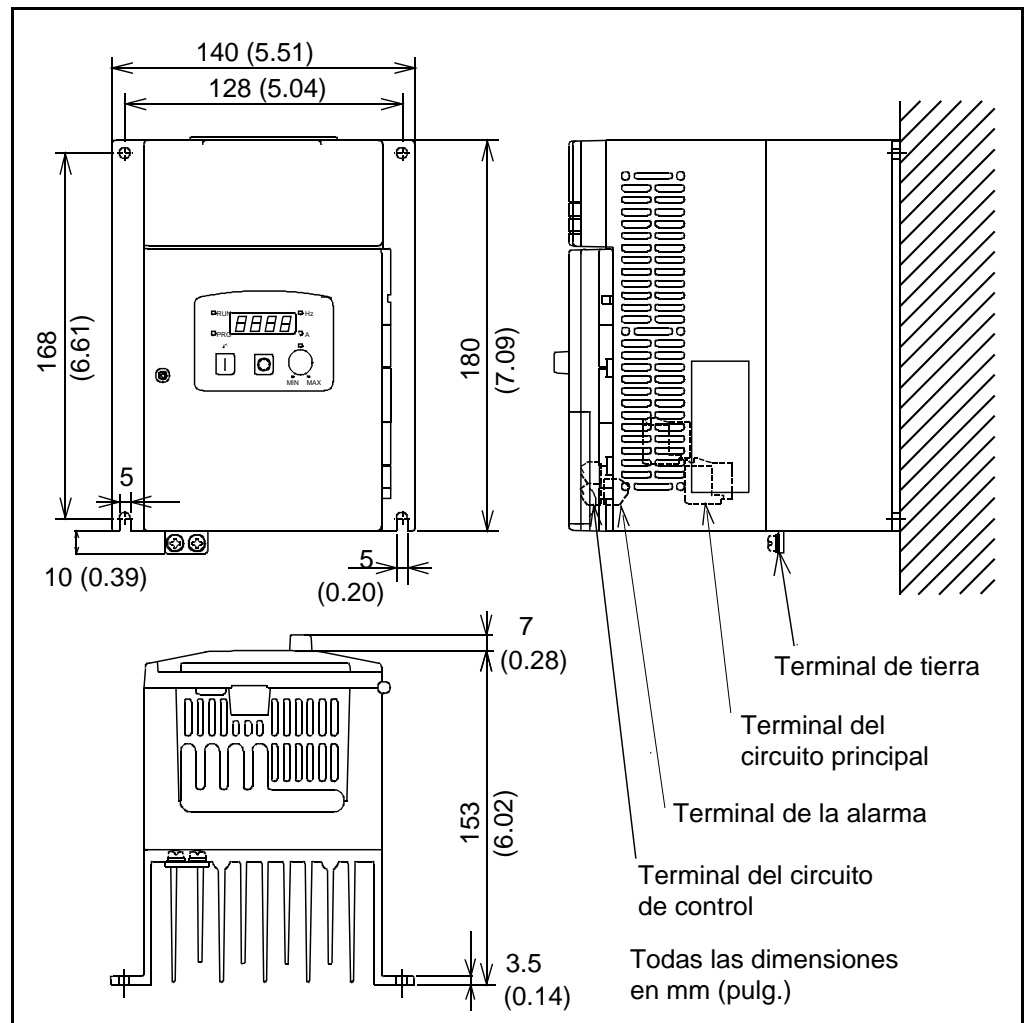
Figura A.3 – Dimensiones del S12-207P1
