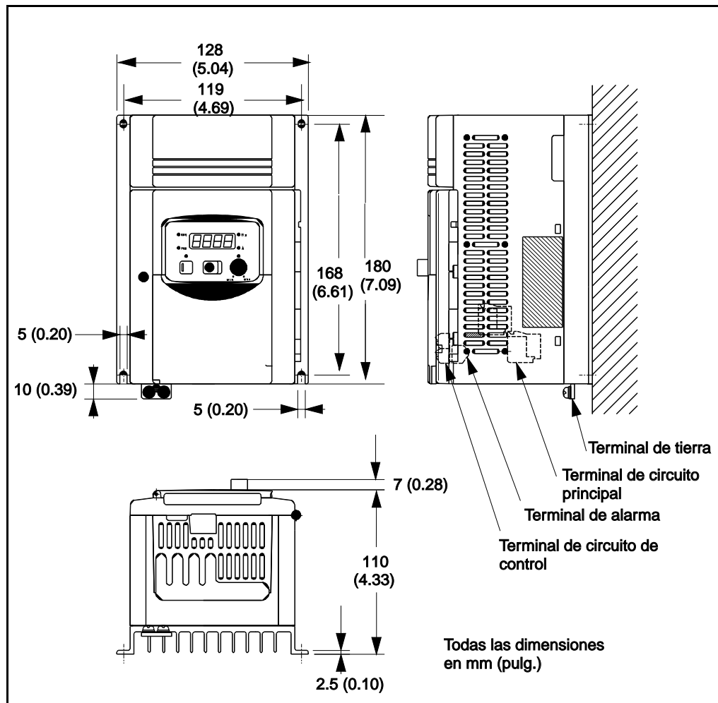
Figura A.6 – Dimensiones del S12-104P0
