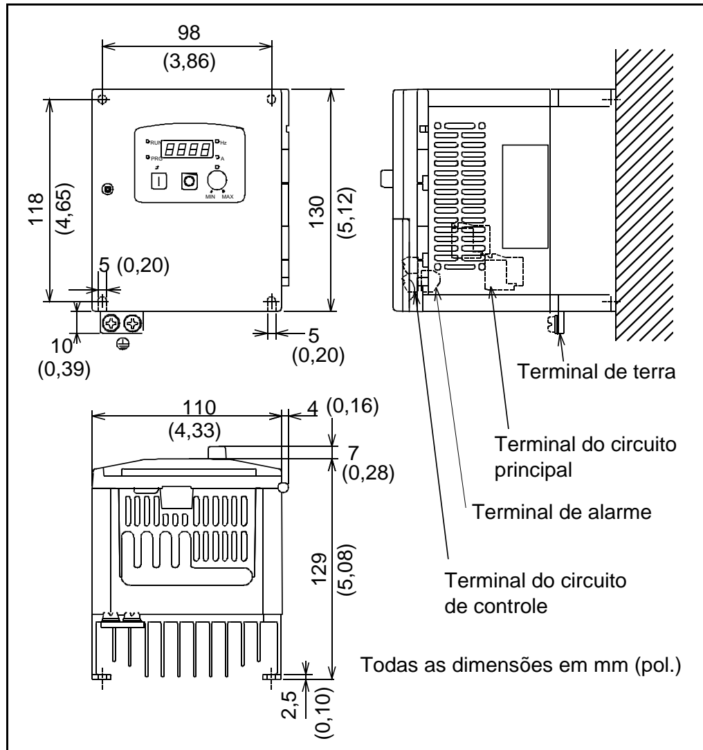
Figura A.2 – Dimensões do S12-204P0 / 205P0 / 401P5
