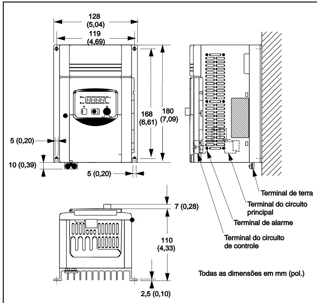
Figura A.6 – Dimensões do S12-104P0
