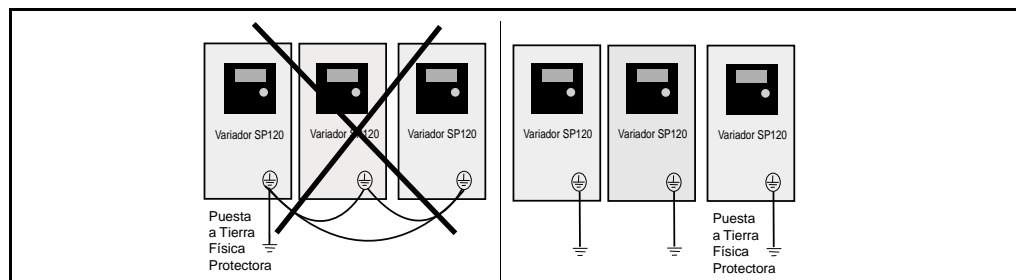
Figura 2.5 – Conexión de puesta a tierra del variador
