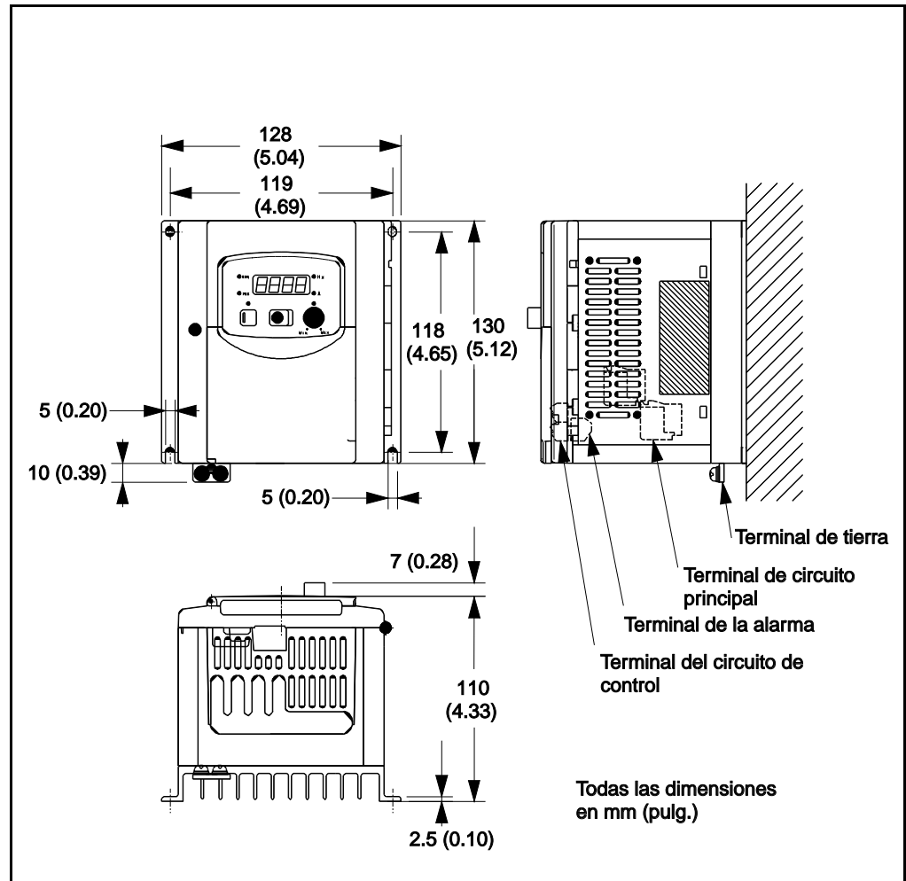
Figura A.5 – Dimensiones del S12-101P4 / 102P6
