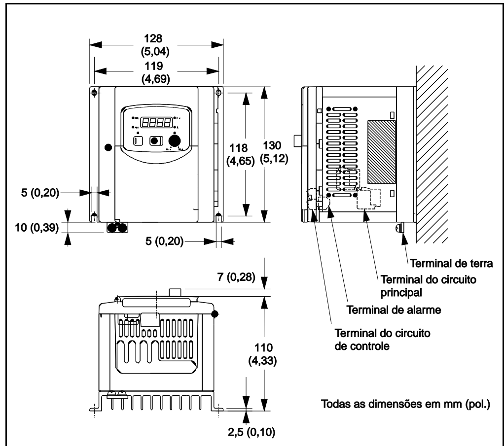
Figura A.5 – Dimensões do S12-101P4 / 102P6
