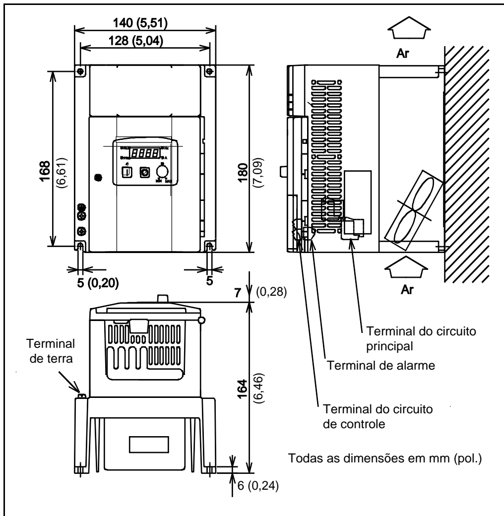
Figura A.4 – Dimensões do S12-20010 / 20015 / 408P6
