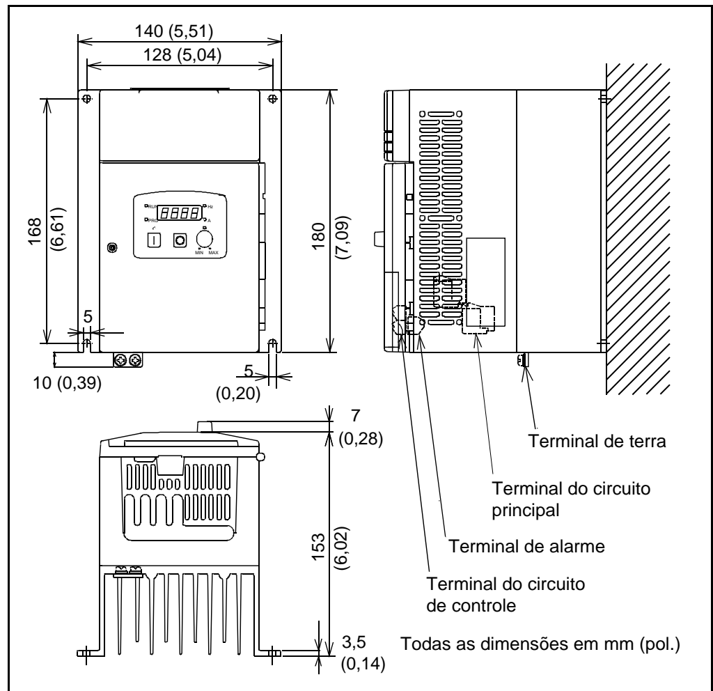
Figura A.3 – Dimensões do S12-207P1
