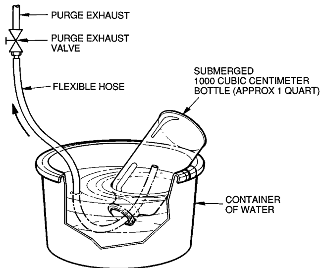
Fig. 27 — Collecting Noncondensables
