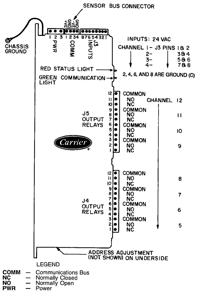
Fig. 21 — Low-Voltage Relay Module (DSIO)
