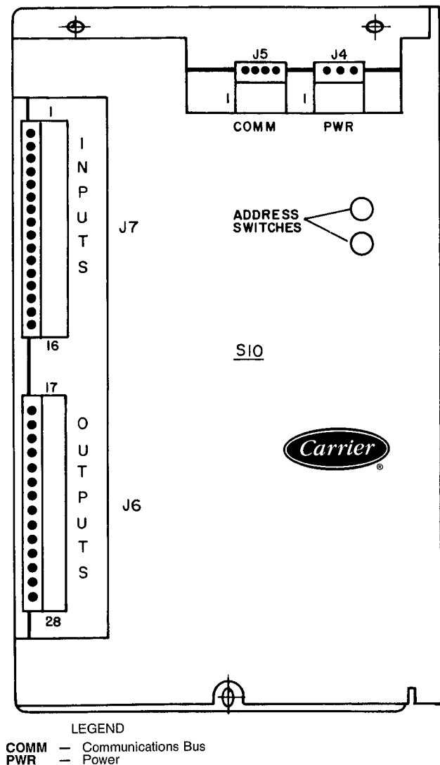
Fig. 22 – 4 In/4 Out Module (SIO)
