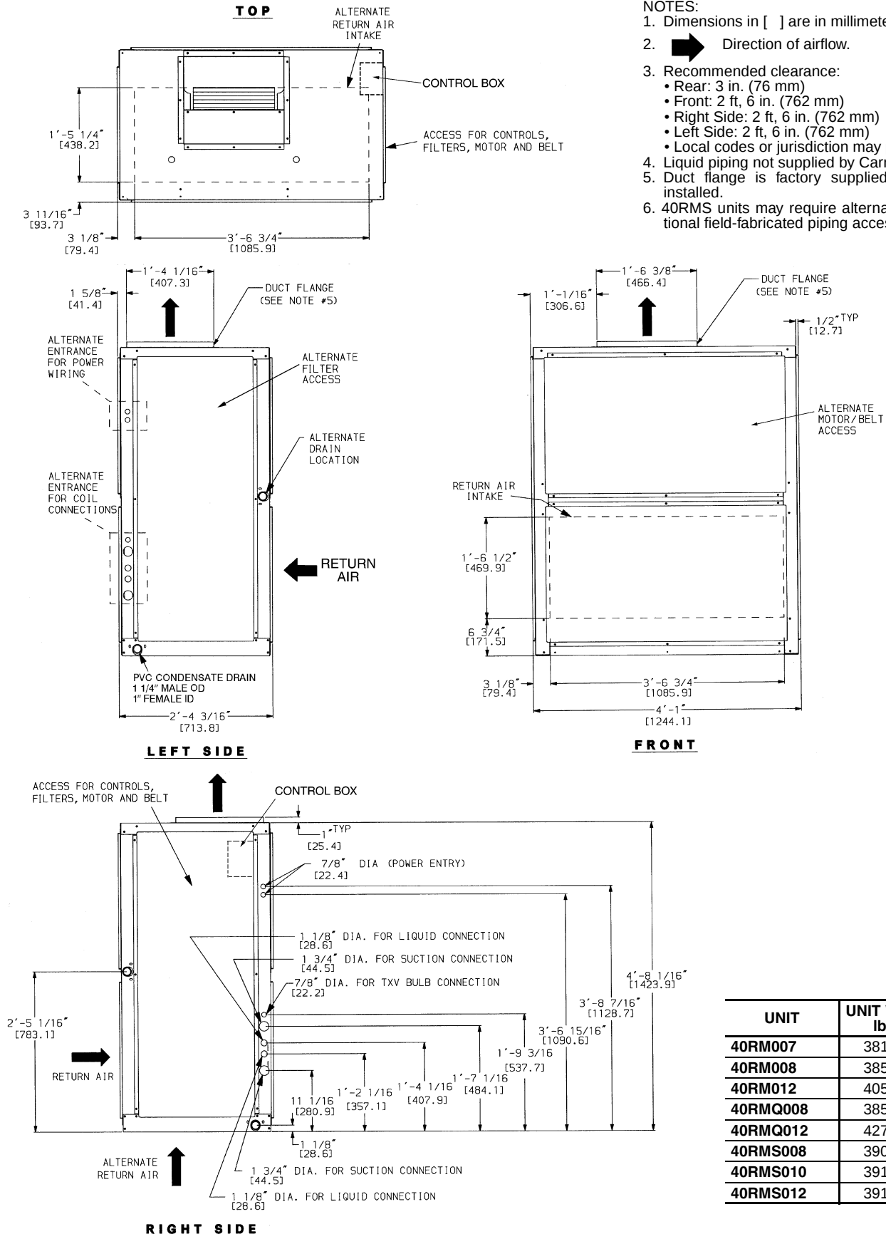
Fig. 1A — Dimensions — Sizes 007-012
