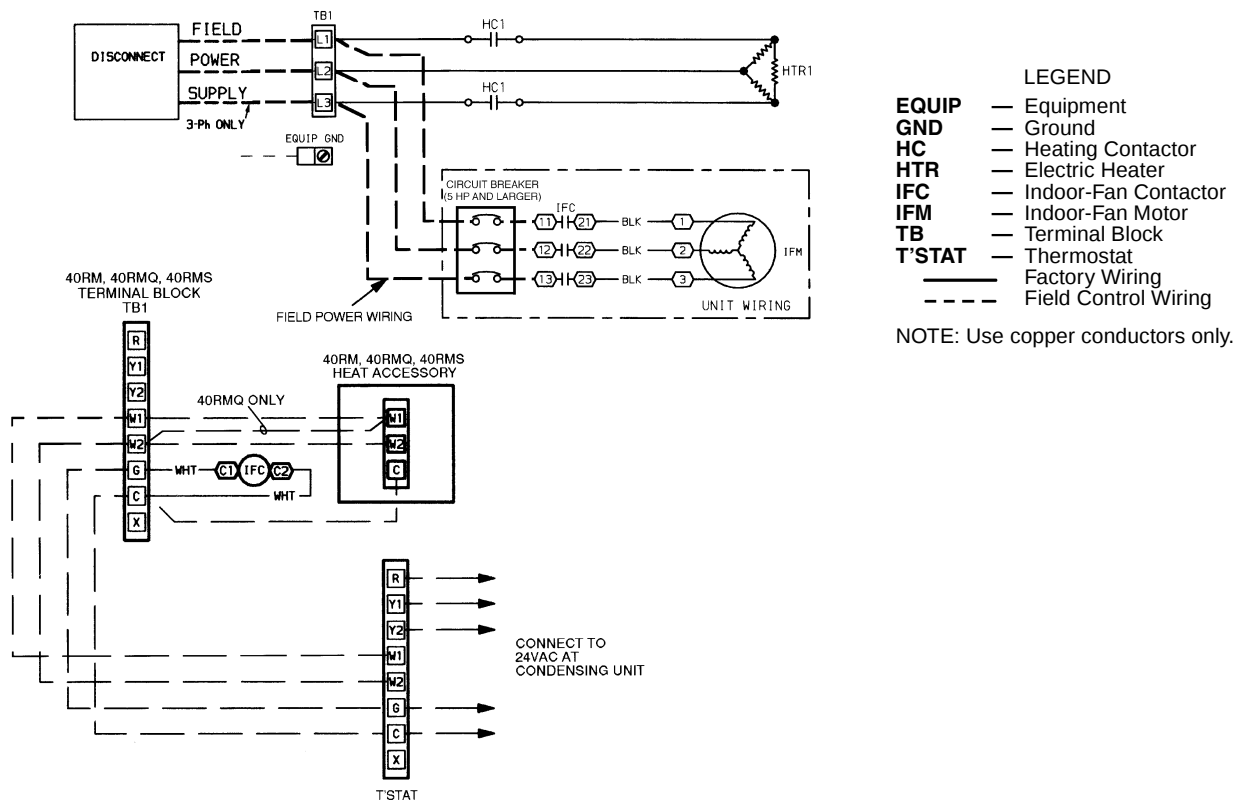
Fig. 17 — Unit Wiring
