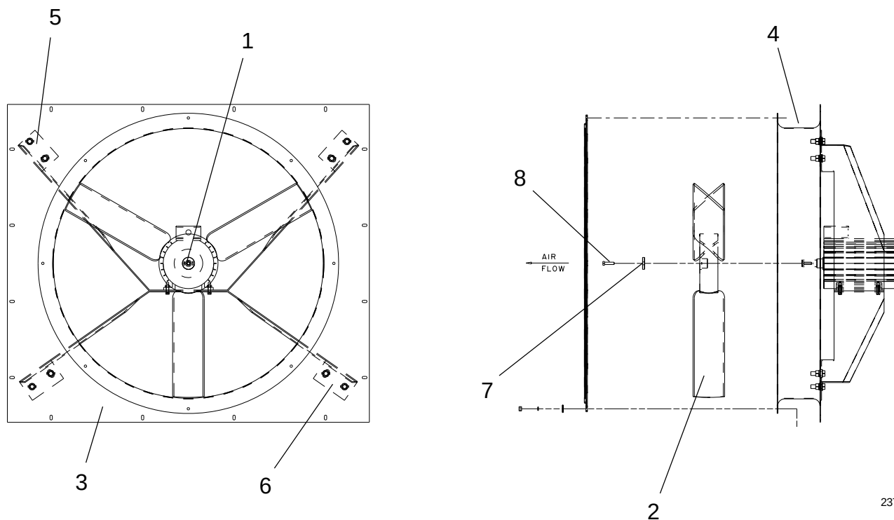
FIG. 4 – FAN COMPONENTS
