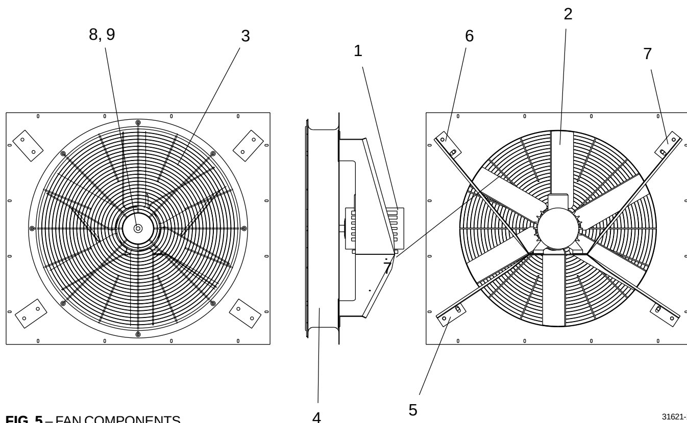
FIG. 5 – FAN COMPONENTS
