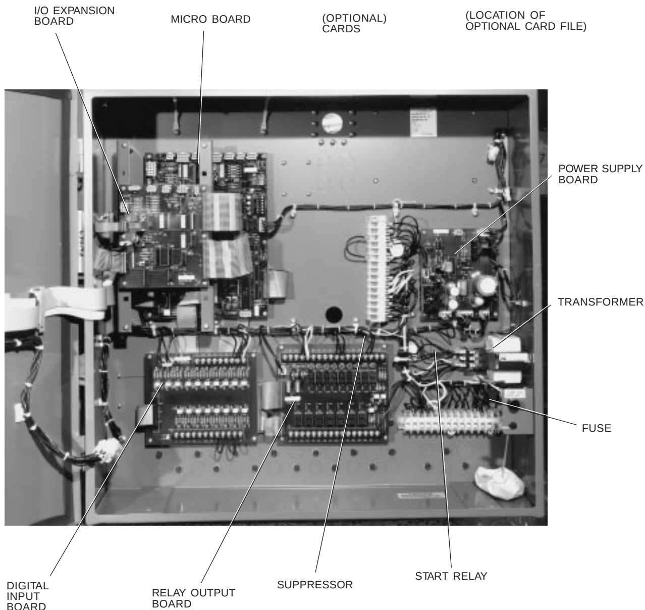
FIG. 2 – MILLENNIUM CONTROL CENTER – DOOR OPEN
