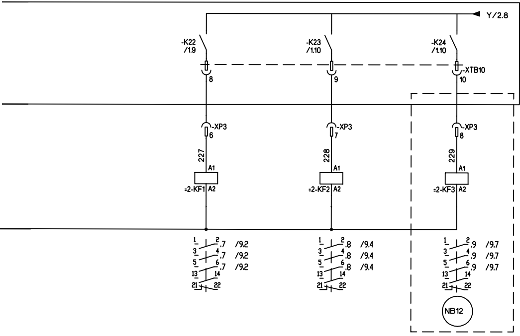
DWG. 3
