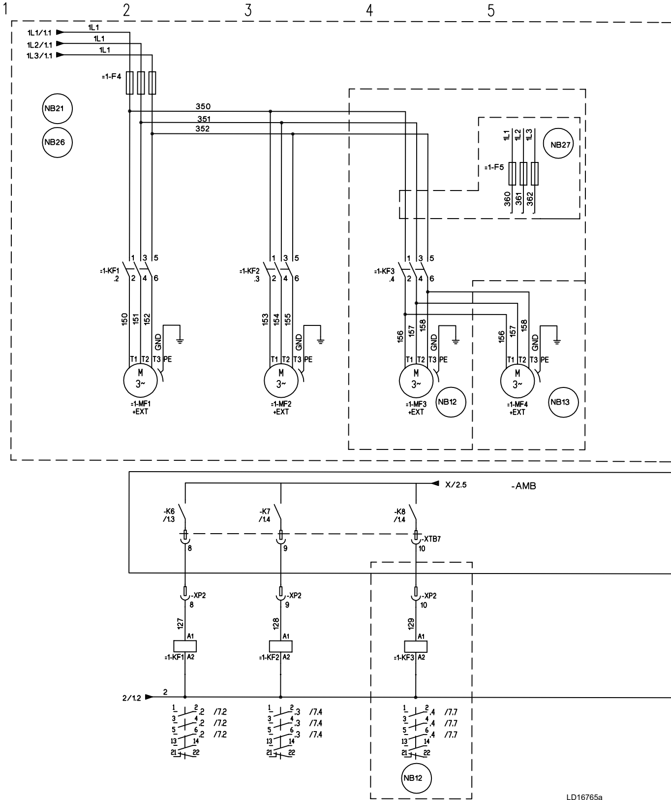
DWG. 3
